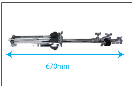
脚部を跳ね上げ式で折りたたむ機構にすることで折り畳み時 670mm のコンパクトさを実現。
